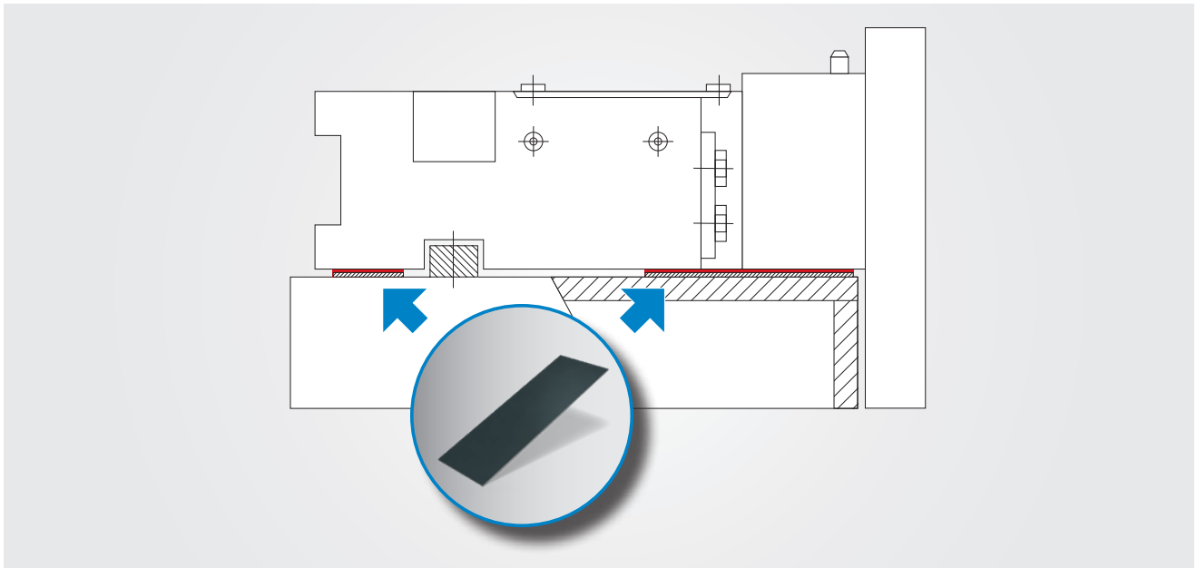
Alojamientos en guías de carro con tiras de deslizamiento Permaglide® PAS ... P180
